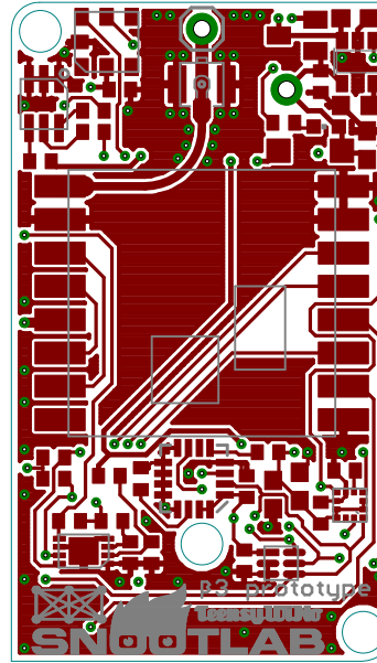
Layer 1 - Top
