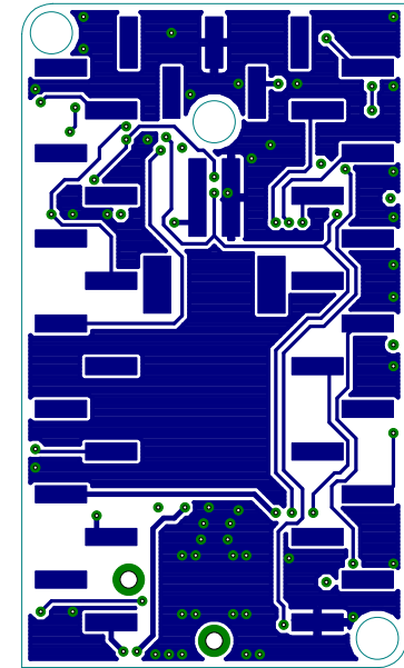
Layer 4 - Bottom
